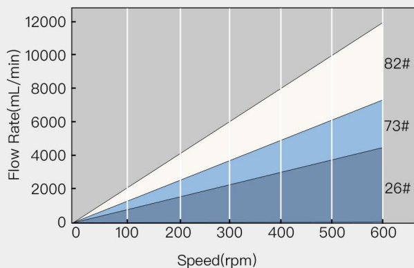
YZ35-II Filling Volume Reference Parameter
