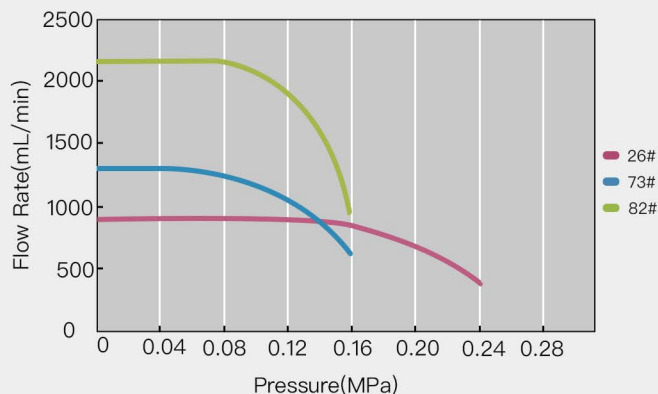
YZ35-II Filling Volume Reference Parameter
